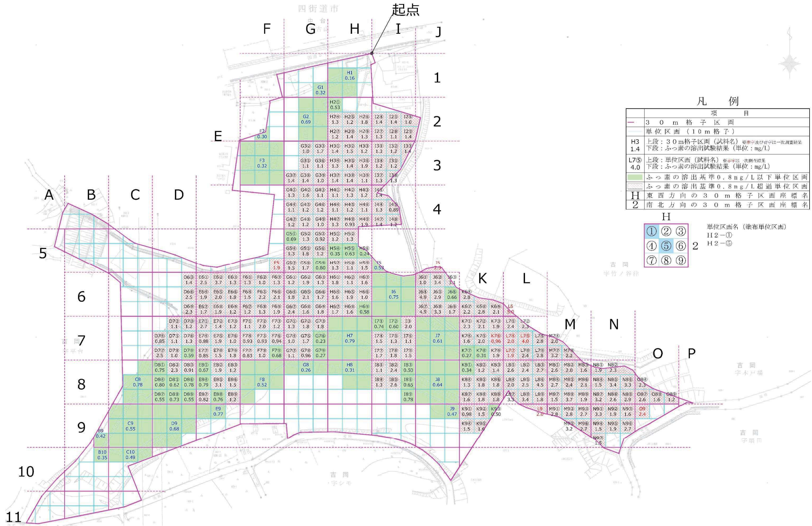
図 3-4 汚染範囲確定調査における土壌溶出試験結果
